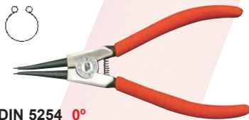
DIN 5254 0°
